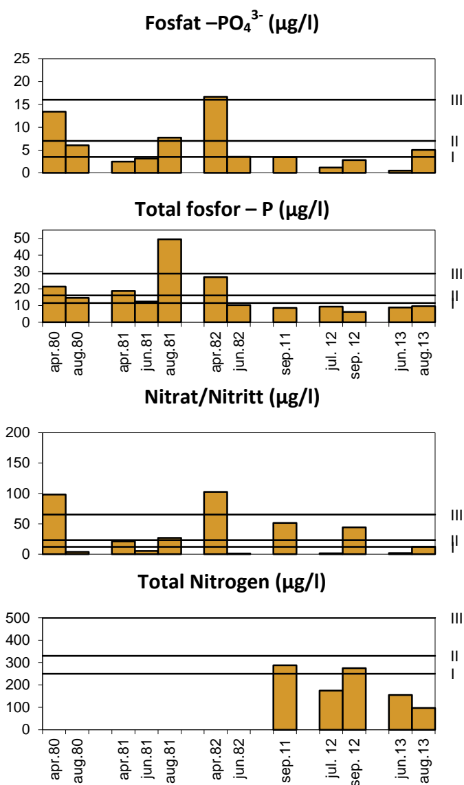
Figur 3.2.8. Gjennomsnittlig konsentrasjon av fosfat, total fosfor, nitrat/nitritt og total mengde nitrogen i prøver fra overflatelaget (0-10 m dyp) ved stasjonen St. 23 (Indre Dolviken) i sommerhalvåret, perioden 1979-2013. Miljødirektoratets tilstandsklasser for sommerhalvåret er markert (I-IV).
