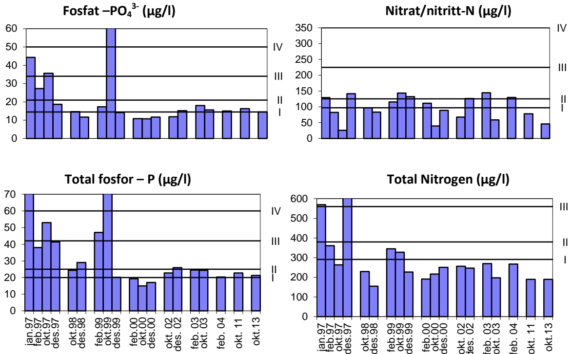
Figur 3.4.12. Gjennomsnittlig konsentrasjon av fosfat, total fosfor, nitrat/nitritt og total mengde nitrogen i prøver fra overflatelaget (0-10 m dyp) ved stasjonen So1 (Indre Soheimsviken) i vinterhalvåret, perioden 1997-2013. Miljødirektoratets tilstandsklasser for vinterhalvåret er markert (I-IV).
