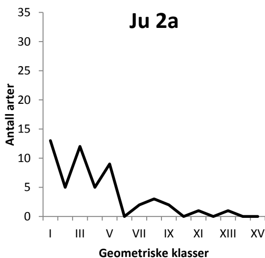
Geometrisk fordeling. Fordeling av arter i geometriske klasser for bunntasjonene i Område 8 for 2013.
