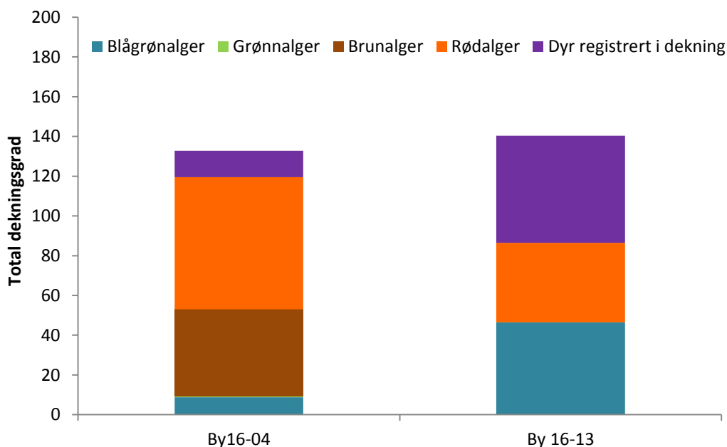
Figur 3.5.14. Total dekningsgrad, fordelt på rød-, brun-, grønnalger, blågrønnalger og dyr registrert som prosent dekning av rutene sammenlignet med tidligere registreringer på stasjonen.
