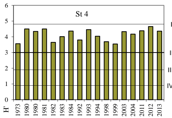
Figur 3.4.43. Utviklingen av artsdiversiteten (H') i sedimentet (basert på sum) fra bunnstasjonene undersøkt i Område 4 i 2013.
