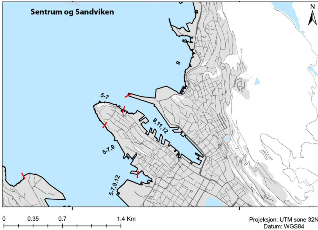
Fig. 3. 4.49. Kartskisse over assosiasjoner av tang, rur og blåskjell i området rundt Centrum /Sandviken etter befarig i juli 2013. Røde streker angir start og stopp for de forskjellige kodene for assosiasjonene. Forklaring av tallkoder er vist i Tabell 3.4.10. Kartkilde: GIS
