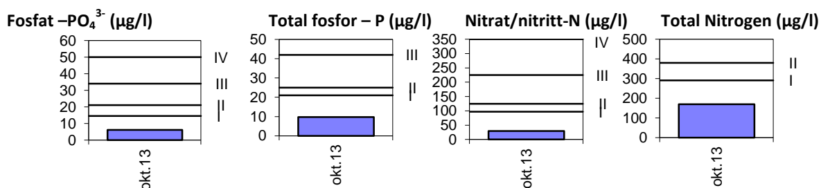
Figur 3.4.15. Gjennomsnittlig konsentrasjon av fosfat, total fosfor, nitrat/nitritt og total mengde nitrogen i prøver fra overflatelaget (0-10 m dyp) ved stasjonen Dra1 (Drageide) i oktober, 2013. Miljødirektoratets tilstandsklasser for vinterhalvåret er markert (I-IV).
