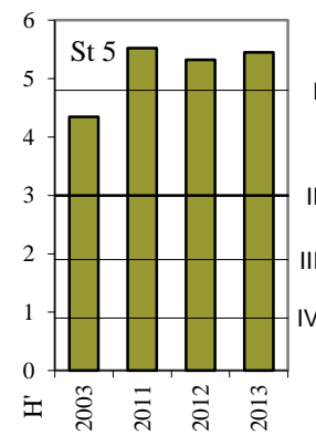
Figur 3.4.43. Utviklingen av artsdiversiteten (H') i sedimentet (basert på sum) fra bunnstasjonene undersøkt i Område 4 i 2013.
