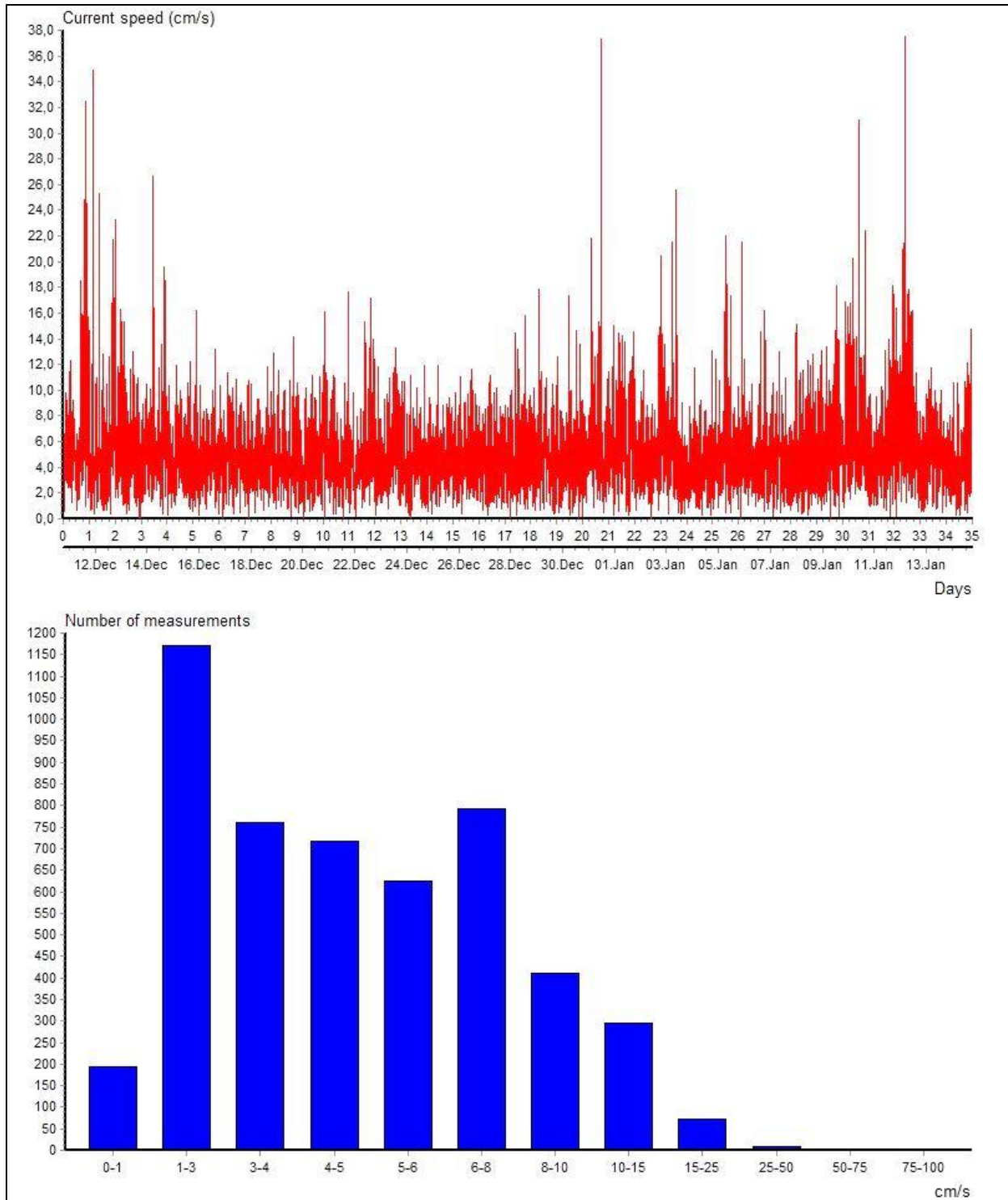
Strømhastigheter nær bunn (51 meters dyp). Strømmålinger på stasjon Kvassneset i perioden 10.desember 2013 til 14.januar 2014.
