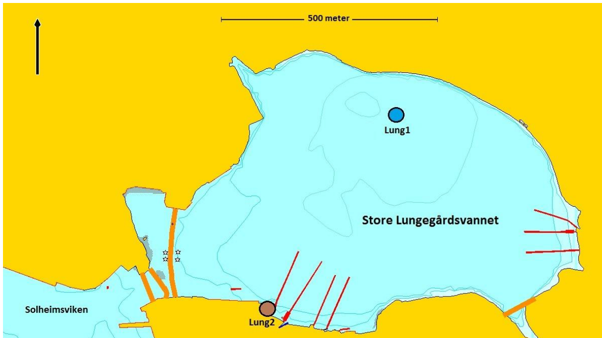
Figur 3.4.2. Kartskisse over prøveinnsamlingsstasjonene i Store Lungegårdsvann 2013 inntegnet. Blå sirkler markerer stasjoner for vannprøvetaking, brune sirkler markerer stasjoner for bunnprøvetaking. Punktets plassering på kartet kan avvike noe fra de nøyaktige GPS-posisjonene angitt i tabell 2.1. Kartkilde: Olex.
