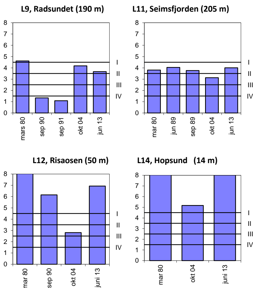
Figur 3.11.7. Oksygenkonsentrasjon i bunnvann for stasjonene i Område 11 i juni. Miljødirektoratets tilstandsklasser for oksygenkonsentrasjon er indikert.
