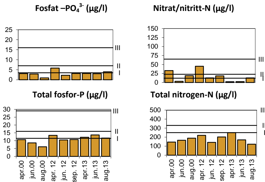
Figur 3.4.24. Gjennomsnittlig konsentrasjon av fosfat, total fosfor, nitrat/nitritt og total mengde nitrogen i prøver fra overflatelaget (0-10 m dyp) ved stasjonen Fag4 (Fagernes) i sommerhalvåret, perioden 2000-2013. Miljødirektoratets tilstandsklasser for sommerhalvåret er markert (I-IV).
