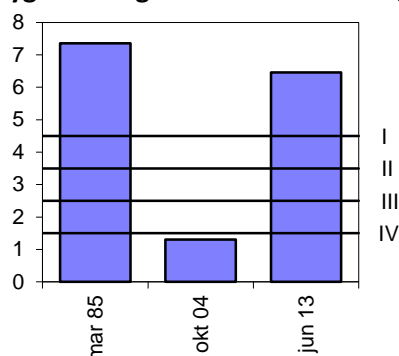
Oksygenmålinger i bunnvann– ml O 2 /l
