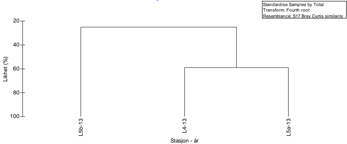
Likhet mellom stasjoner uttrykt gjennom en clusteranalyse av artslistene fra stasjonene i Område 9 , 2013.
