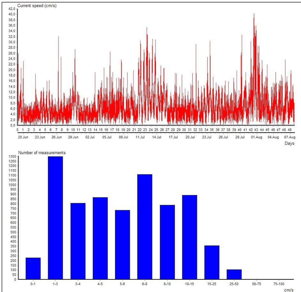
Strømhastigheter i overflaten (9 meters dyp). Strømmålinger på stasjon Kvassneset i perioden 18.juni 2013 til 7. august 2013.
