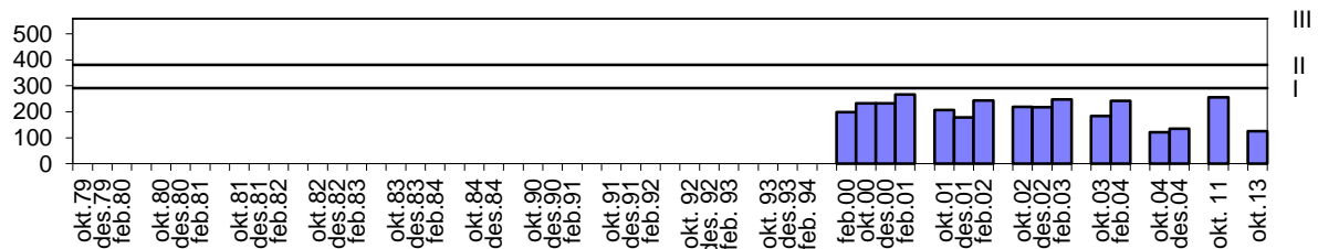
Figur 3.2.3. Gjennomsnittlig konsentrasjon av nitrat/nitritt, fosfat, total fosfor, og total mengde nitrogen i prøver fra overflatelaget (0-10 m dyp) ved stasjonen St. 18 (Ytre Dolviken) i vinterhalvåret, perioden 1979-2013. Miljødirektoratets tilstandsklasser for vinterhalvåret er markert (I-IV).
