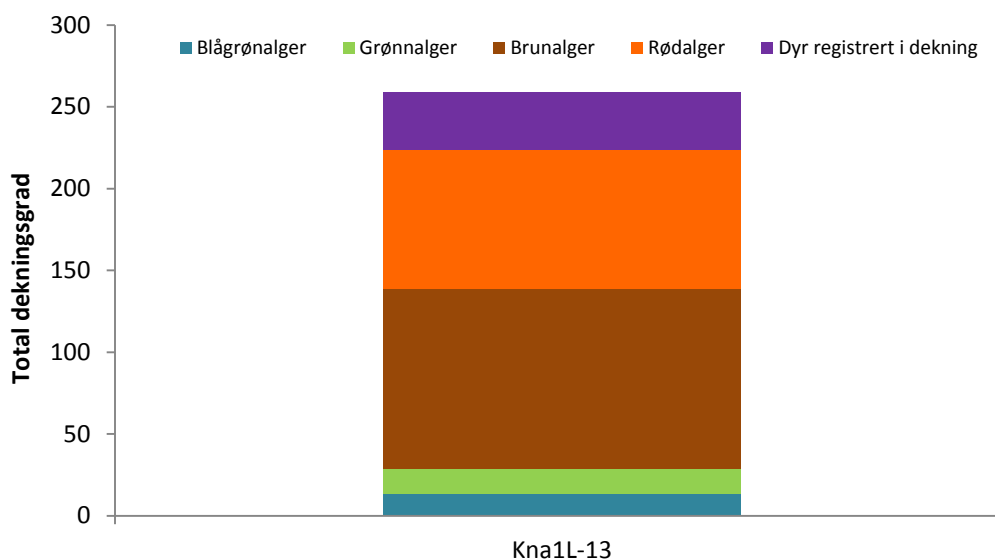
Figur 3.1.19: Total dekningsgrad, fordelt på rød-, brun-, grønner, blågrønner og dyr registrert som prosent dekning av rutene på stasjonen Kna1L, 2013.
