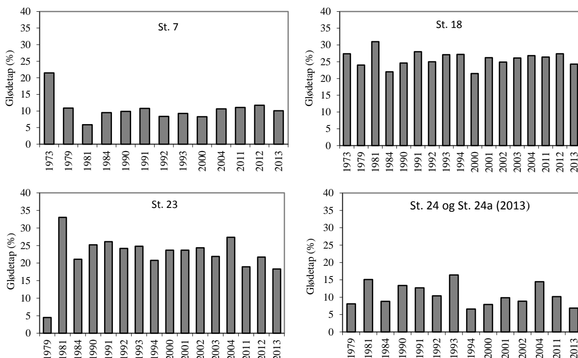
Figur 3.2.14. Utviklingen av organisk innhold i sedimentet (% glødetap) ved stasjonene i Område 2.
