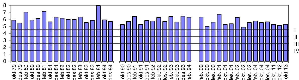
Figur 3.2.10 Oksygenkonsentrasjon i vintermånedene ved 80 m dyp ved stasjonen St. 7 (Grimstadfjorden). Miljødirektoratets Tilstandsklasser for oksygenkonsentrasjon i bunnvann er indikert (Veileder 02:2013).
