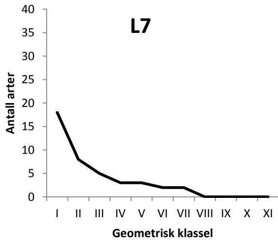
Geometrisk fordeling. Fordeling av arter i geometriske klasser for bunnstasjonene i Område 10 for 2013.
