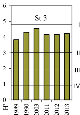
Figur 3.4.43. Utviklingen av artsdiversiteten (H') i sedimentet (basert på sum) fra bunnstasjonene undersøkt i Område 4 i 2013.
