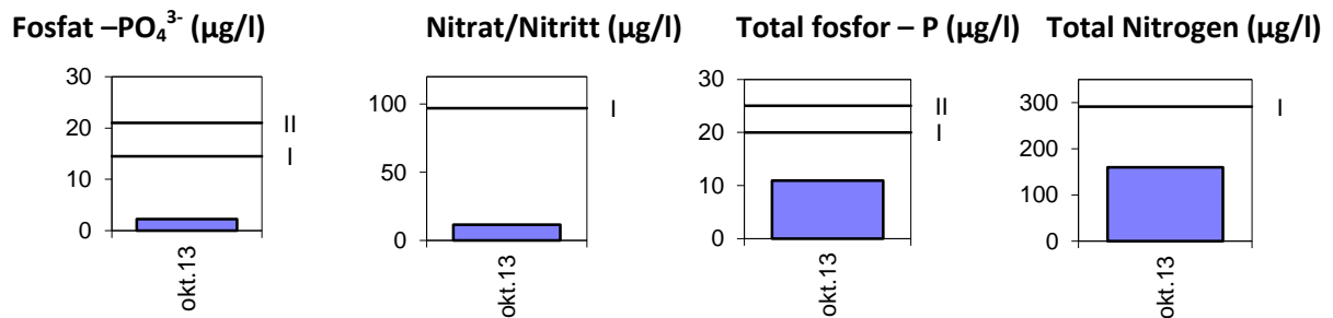
Figur 3.8.3. Gjennomsnittlig konsentrasjon av fosfat, total fosfor, nitrat/nitritt og total mengde nitrogen i prøver fra overflatelaget (0-10 m dyp) ved stasjonen Ju2a (Juvik) i vinterhalvåret i oktober 2013. Miljødirektoratets tilstandsklasser for vinterhalvåret er markert (I-IV).
