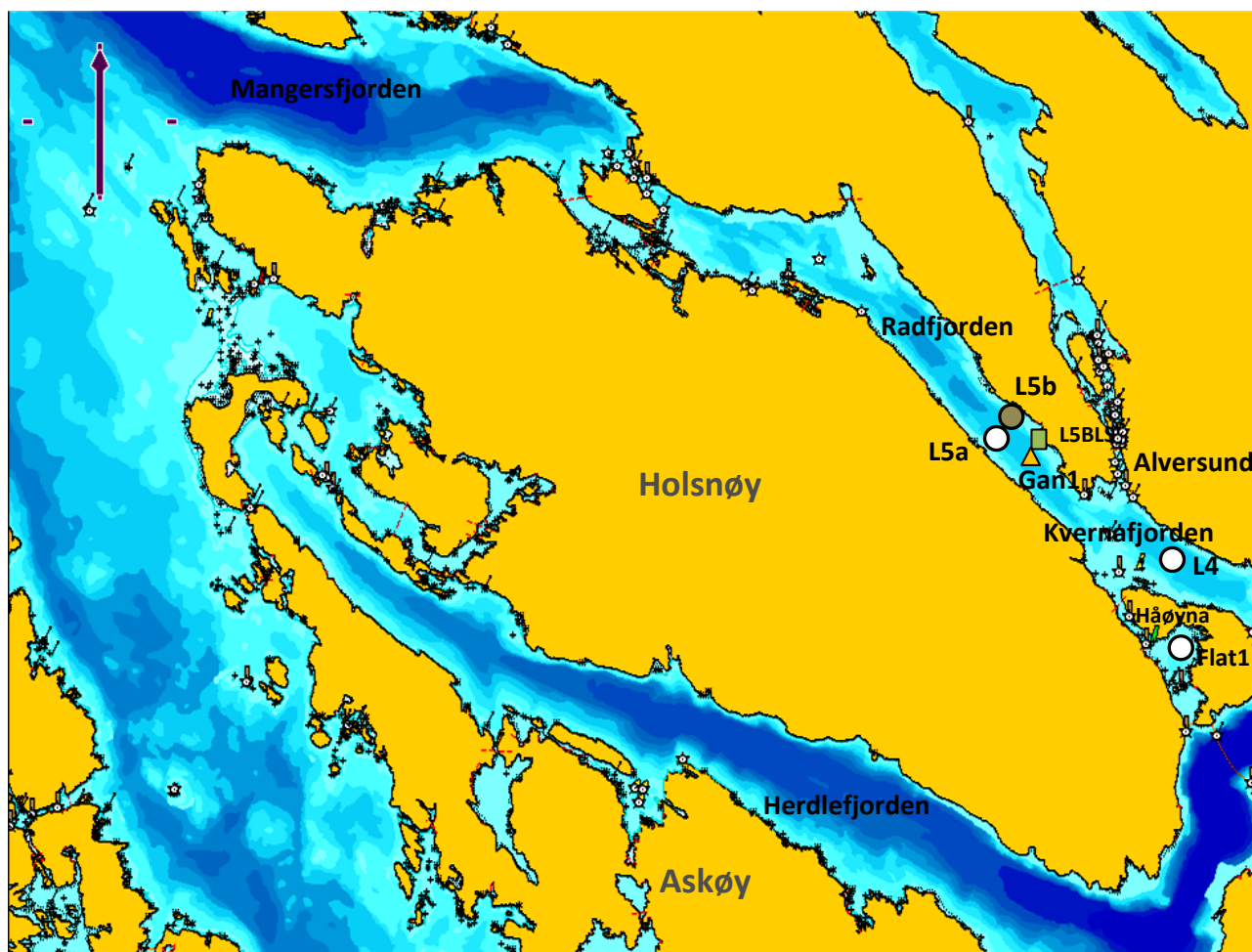
Figur 3.9.1. Kartskisse over Område 9 med prøveinnsamlingsstasjonene inntegnet. Hvite sirkler markerer stasjoner med både bunn- og vannprøver, mørkeblå stasjoner kun vannprøver, mens brune stasjoner markerer kun bunnprøver. Fjæresonestasjonen (semikvantitativ undersøkelse og innsamling av biota) L5BLS er merket med grønn firkant. Strømmålinger merket med oransje trekant. Punktets plassering på kartet kan avvike noe fra de nøyaktige GPS-posisjonene angitt i tabell 2.1. Kartkilde: Olex.
