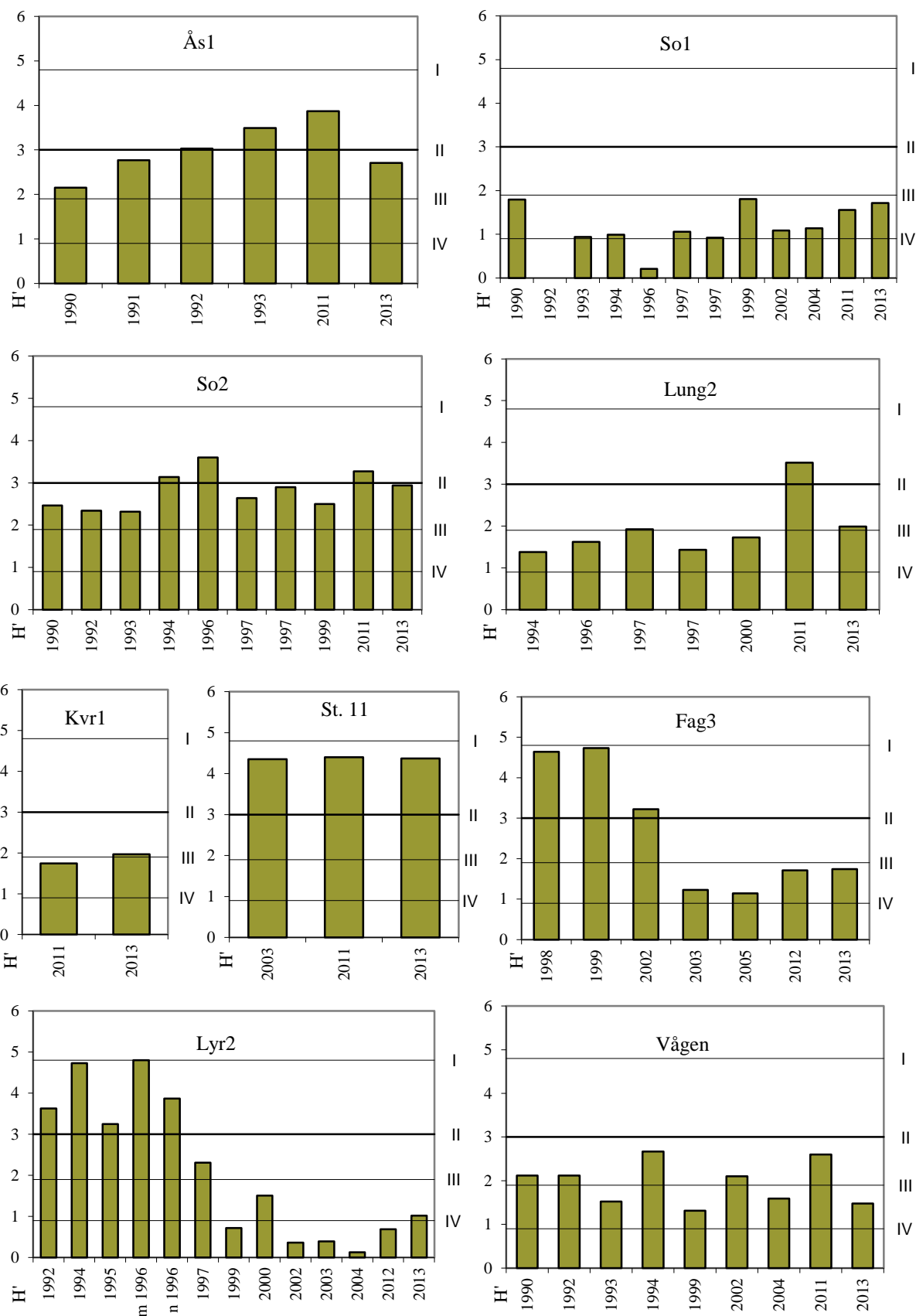
Figur 3.4.43. Forts. Utviklingen av artsdiversiteten (H') i sedimentet (basert på sum) fra bunnstasjonene undersøkt i Område 4 i 2013.
