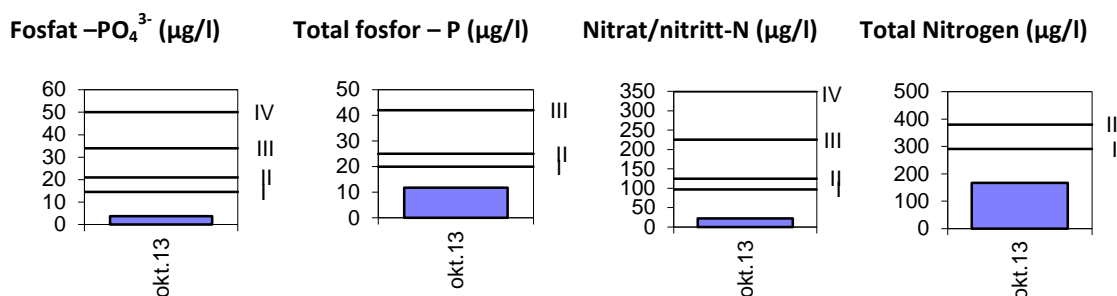
Figur 3.4.16. Gjennomsnittlig konsentrasjon av fosfat, total fosfor, nitrat/nitritt og total mengde nitrogen i prøver fra overflatelaget (0-10 m dyp) ved stasjonen Klep1 (Kleppestø) i oktober 2013. Miljødirektoratets tilstandsklasser for vinterhalvåret er markert (I-IV).
