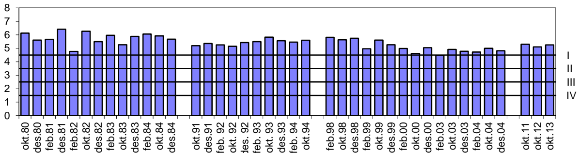
Figur 3.4.34. Oksygenkonsentrasjon i vintermånedene på 330 m dyp ved stasjonen St. 4 (Midtre Byfjorden) i perioden 1980-2013. Miljødirektoratets Tilstandsklasser for oksygenkonsentrasjon i bunnvann er vist (Veileder 02:2013).
