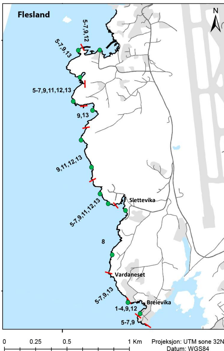
Fig. 3.3.10. Kartskisse over assosiasjoner av tang, rur og blåskjell i området rundt Flesland etter befaring i juli 2013. Røde streker angir start og stopp for de forskjellige kodene for assosiasjonene. Forklaring av tallkoder er vist i Tabell 3.3.6. Grønne sirkler angir fotolokasjoner (FL1-FL13 fra sør mot nord). Kartkilde: GIS
