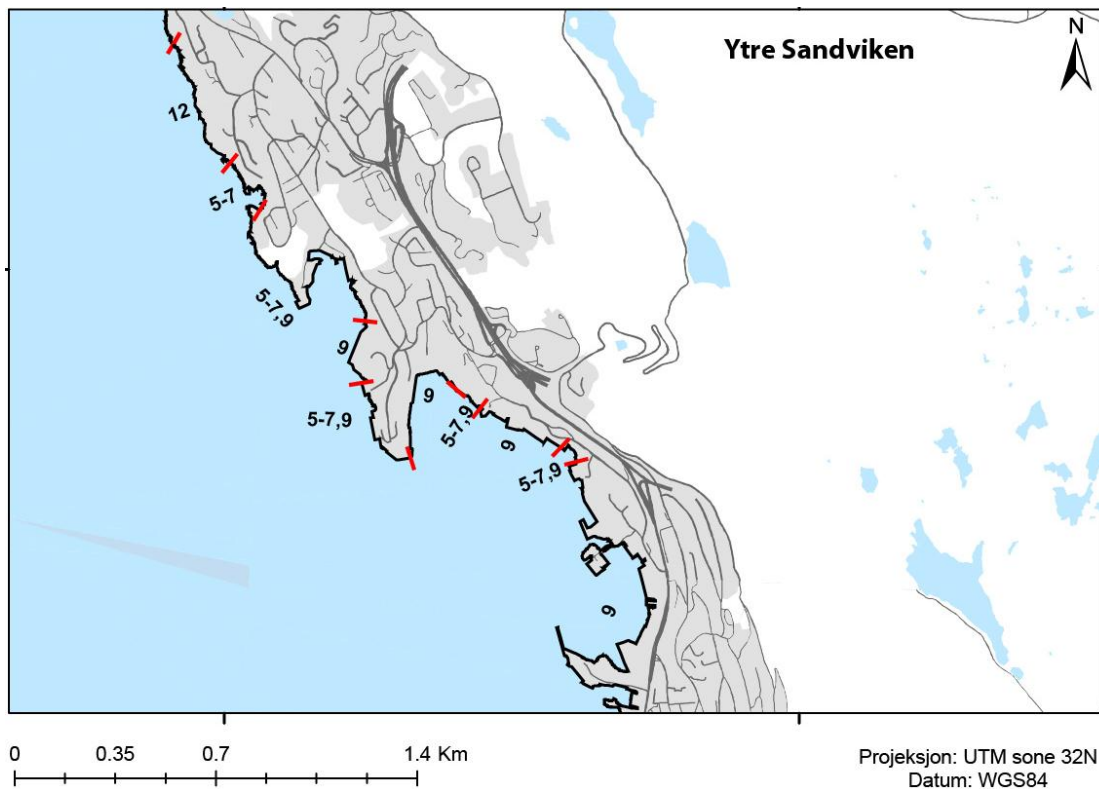
Fig. 3. 4.50. Kartskisse over assosiasjoner av tang, rur og blåskjell i området rundt Ytre Sandviken etter befarig i juli 2013. Røde streker angir start og stopp for de forskjellige kodene for assosiasjonene. Forklaring av tallkoder er vist i Tabell 3.4.10. Kartkilde: GIS
